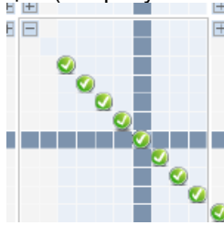
Рисунок 3.3 - Настройка матрицы
