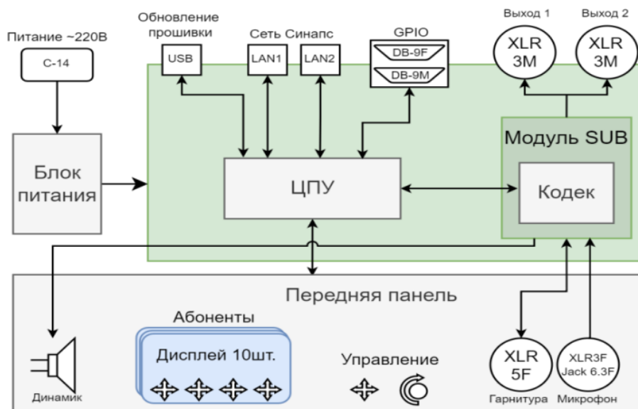
Рисунок 2.1 - Блок TP-840. Структурная схема
