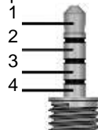
Рисунок 2.11 - Цоколёвка разъема Mini-Jack 3.5mm 4pin
