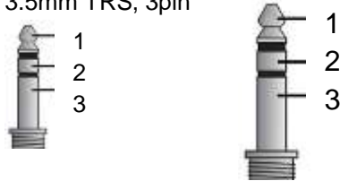
Рисунок 2.6 - Цоколёвка разъёма Jack 3.5mm TRS, 3pin
