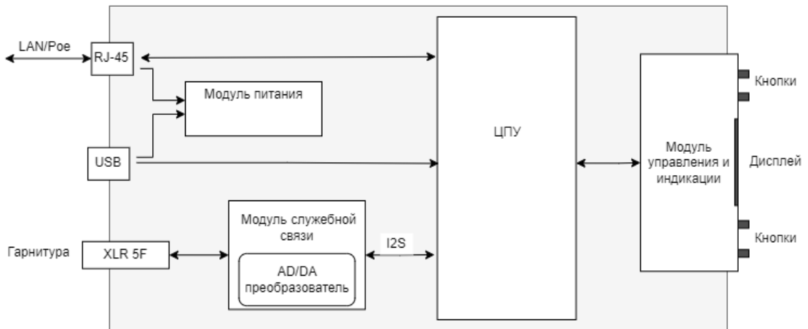
Рисунок 2.1 - TP-803. Схема структурная
