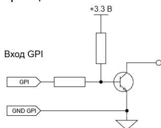
Рисунок 2.5 - Вход GPI, схема принципиальная.
