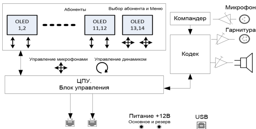
Рисунок 2.1 - Блок TP-812. Структурная схема
