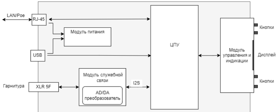
Рисунок 2.1 - TP-803. Схема структурная
