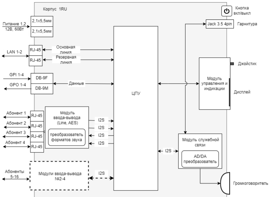
Рисунок 2.1 – TP-804. Схема структурная, модули Line и AES
