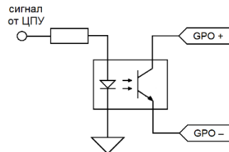
Рисунок 4.1 – Выход GPO, схема принципиальная
