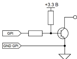
Рисунок 4.2 – Вход GPI, схема принципиальная
