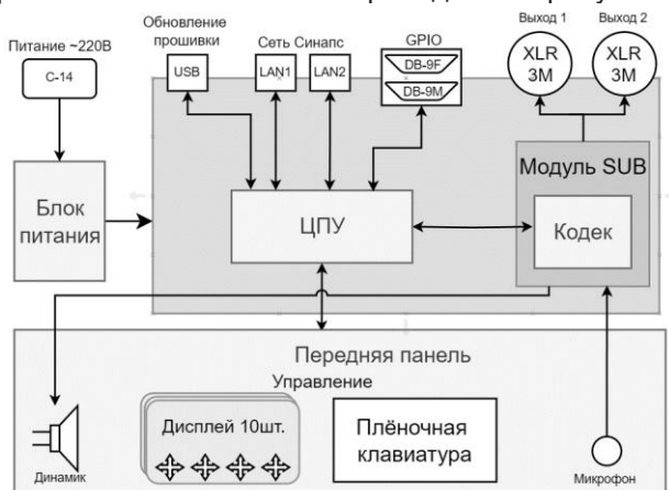
Рисунок 2.1 - Блок TP-832. Структурная схема
