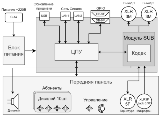
Рисунок 2.1 - Блок TP-840. Структурная схема
