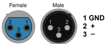
Рисунок 4.2 – Разъёмы XLR F и XLR M
