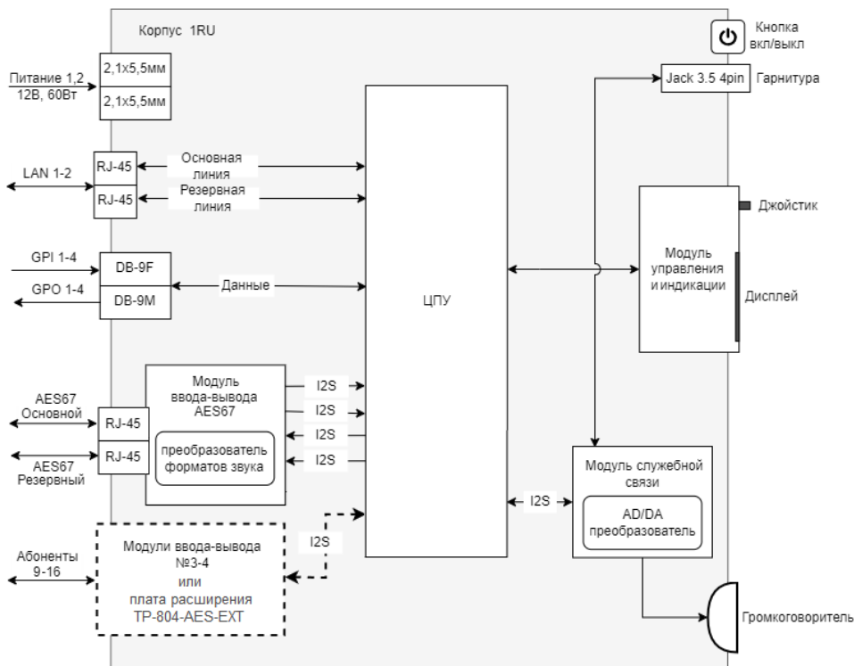
Рисунок 2.1 – TP-804 с модулем TP-804-AES67
