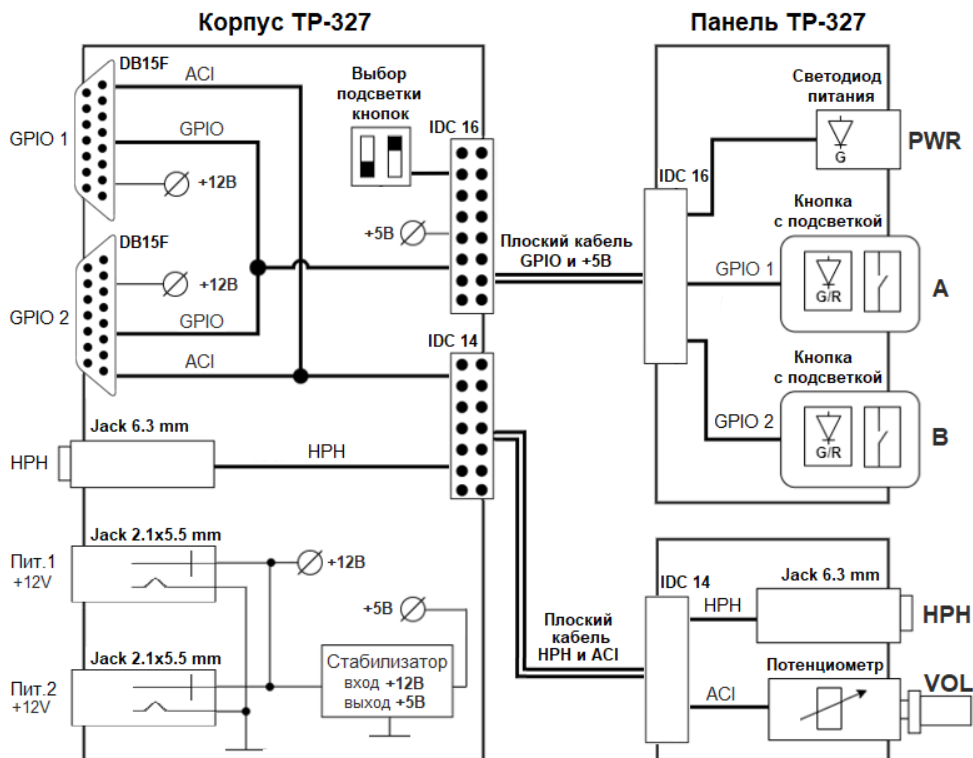
Рисунок 2.2 - TP-327. Схема структурная
