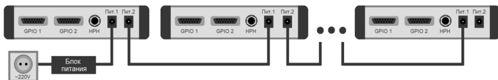
Рисунок 2.5 – Схема подключения питания нескольких TP-327
