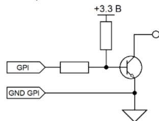
Рисунок 3.4 – Вход GPI, схема принципиальная
