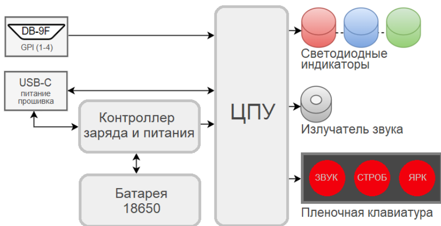
Рисунок 3.1 - Структурная схема Блока
