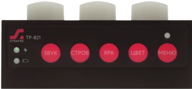
Рисунок 3.2 - Блок TP-821. Передняя панель
