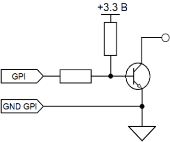
Рисунок 2.4 - Вход GPI, схема принципиальная
