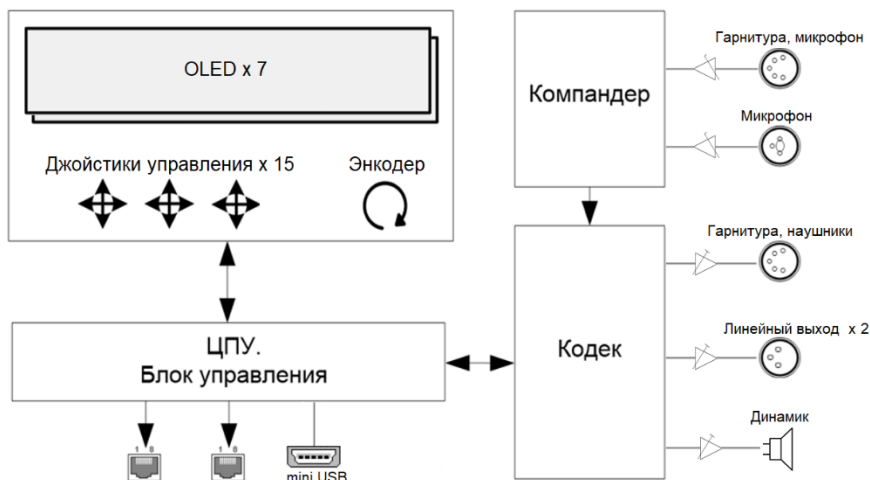
Рисунок 2.1 - Блок TP-812. Структурная схема
