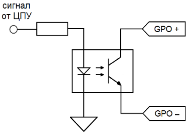
Рисунок 2.5 - Выход GPO, схема принципиальная
