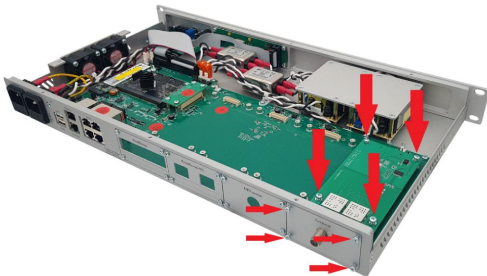
Рисунок 10 – Установка модуля
