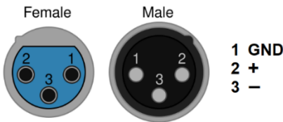
Рисунок 5 - Цоколёвка разъемов XLR
