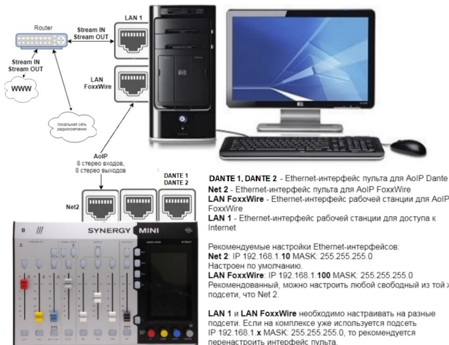
Рисунок 6 - Настройки сетевых интерфейсов
