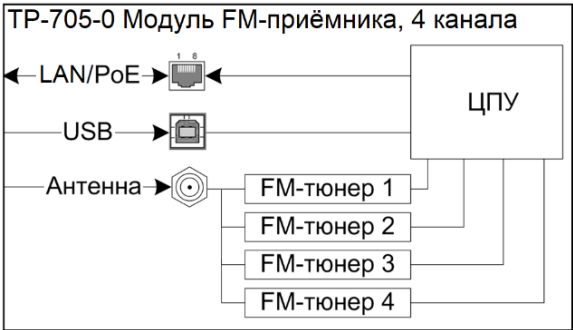
Рисунок 2.1 – Структурная схема модуля TP-705-0
