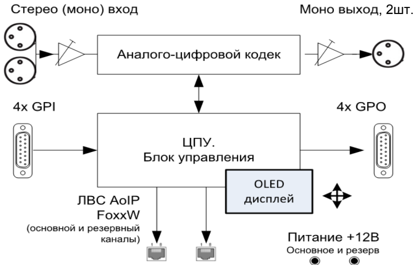
Рисунок 4.1 - TP-801. Схема структурная
