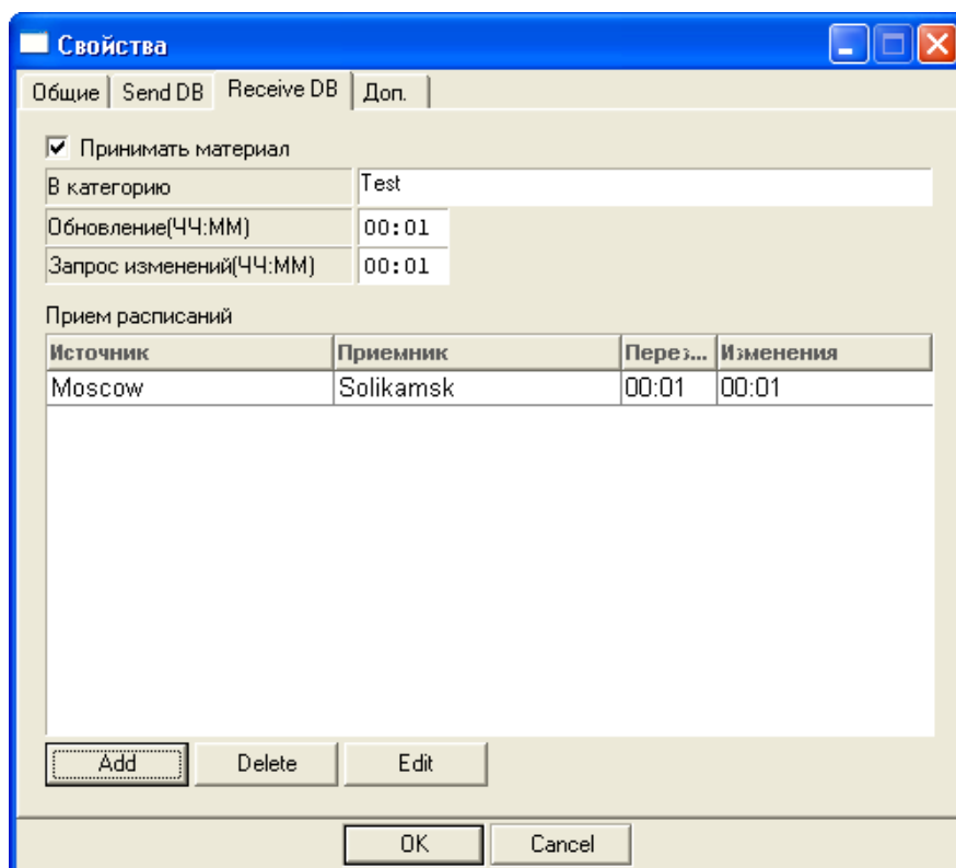
Рис. 8. Окно Свойства соединения закладка Receive DB
