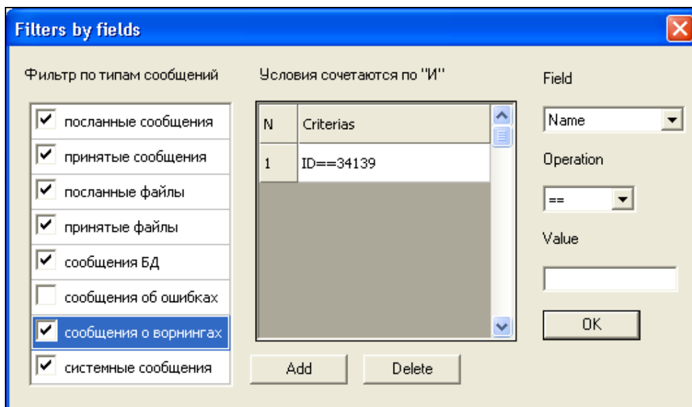
Рис. 15. Диалоговое окно Фильтрации по полям
