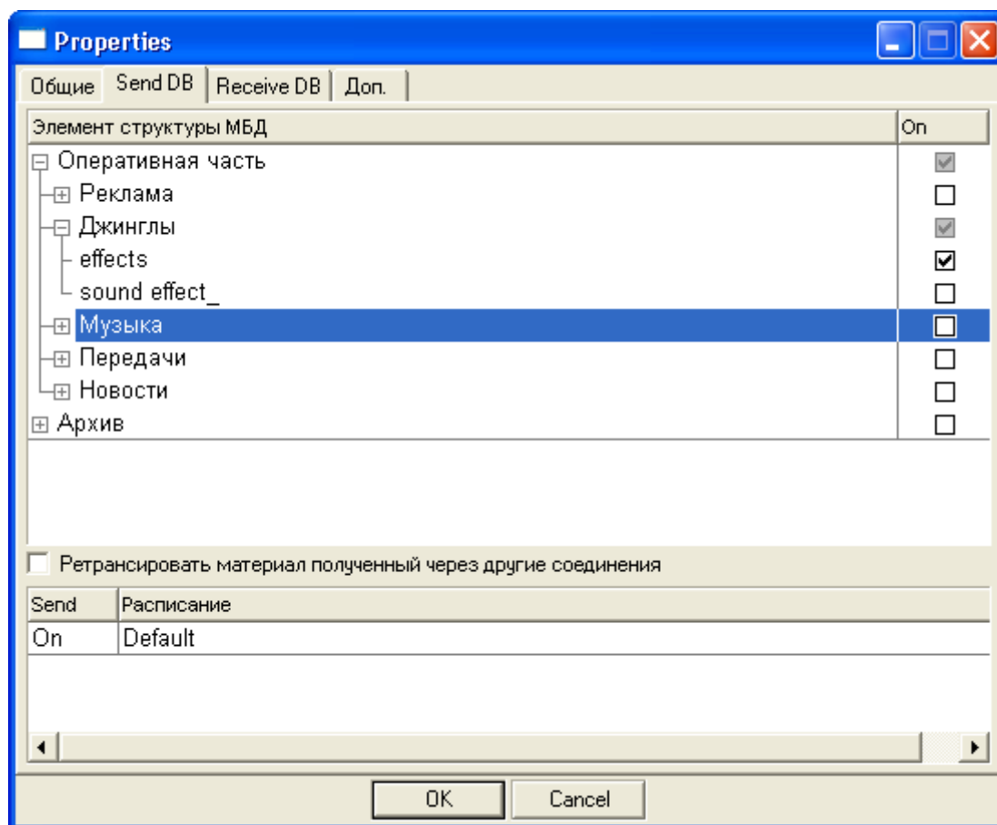
Рис. 5. Окно Свойства соединения закладка Send
