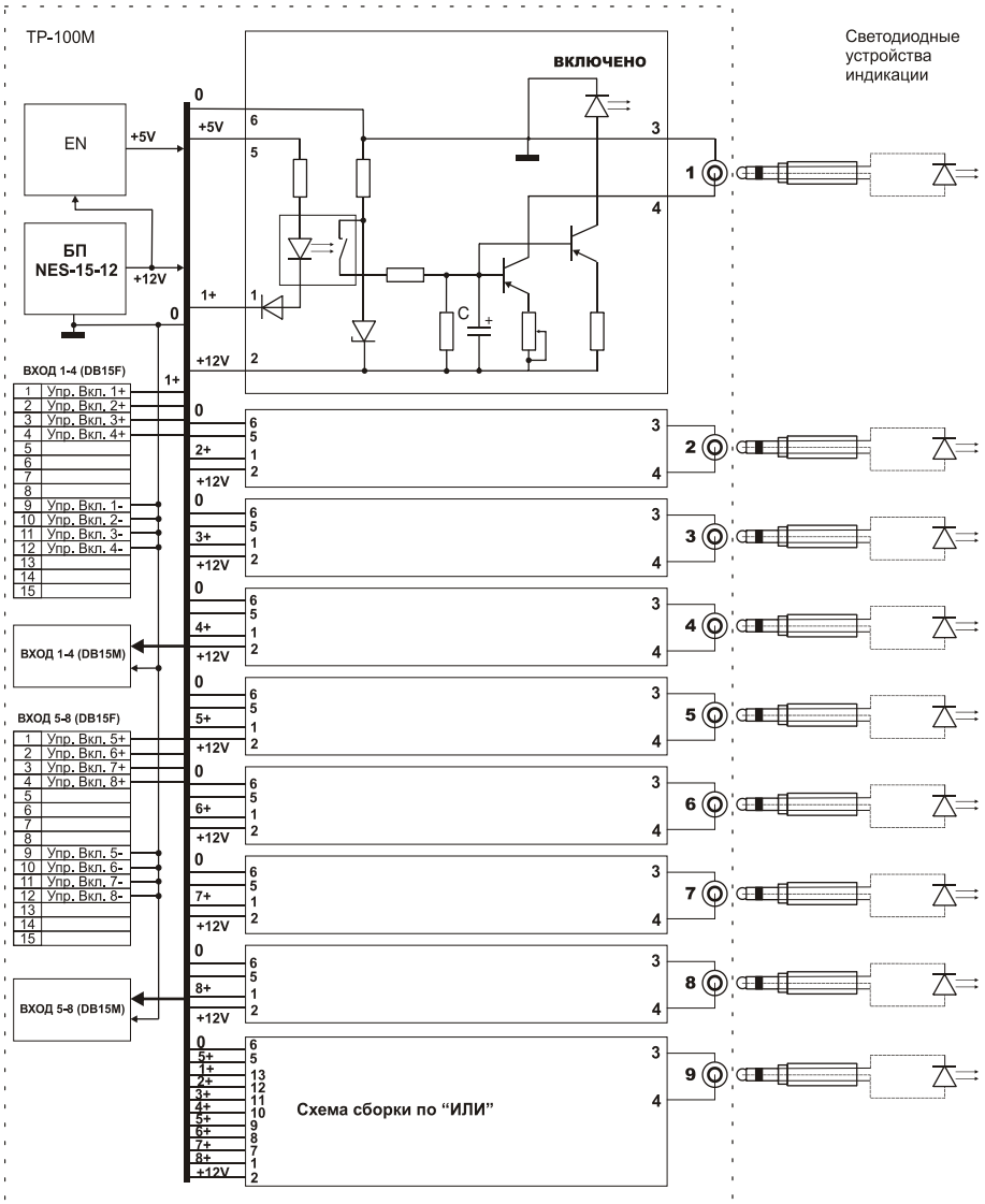
Рис. 1. Структурная схема блока TP-100M
